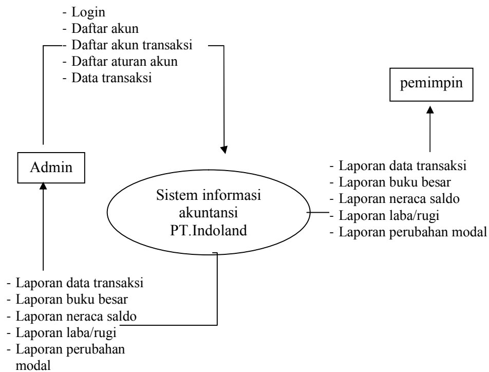
Gambar 1 DFD Level Konteks Sistem Informasi Akuntansi
