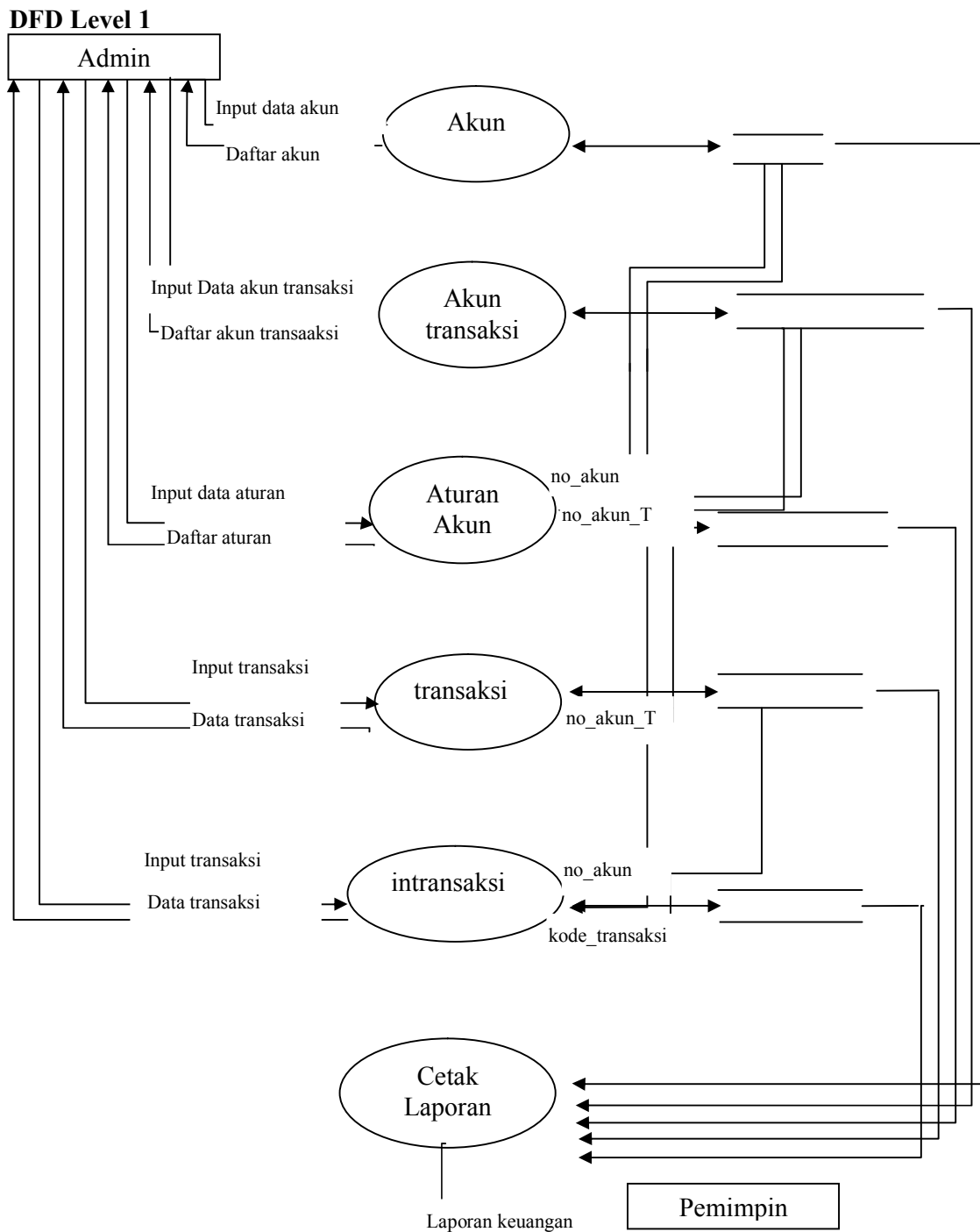
Gambar 3.7 DFD Level 1 Sistem Informasi Akuntansi
