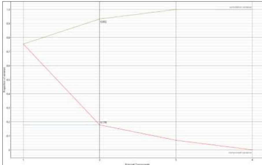
Gambar 6. Grafik hasil analisis komponen utama
