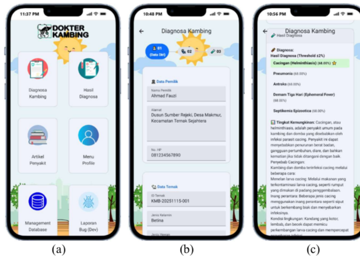
Figure 4. Tangkapan Layar: (a) Halaman Utama, (b) Input Data Diagnosa, (c) Hasil Diagnosa
