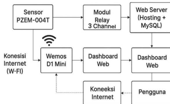
Gambar 2. Blok Diagram Alat
