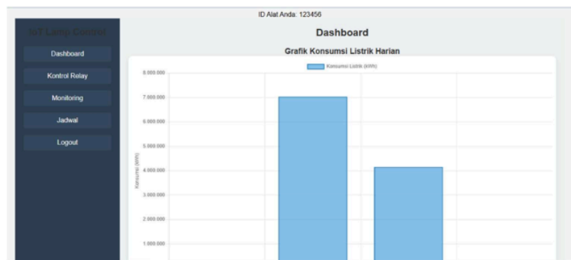
Gambar 7. Implementasi Tampilan Pada Halaman Dashboard
