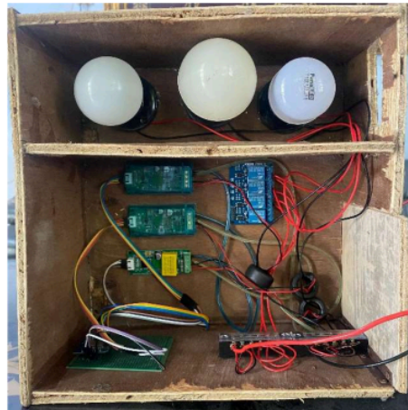
Gambar 12. Alat Saat Dipasang untuk Pengujian Lampu
