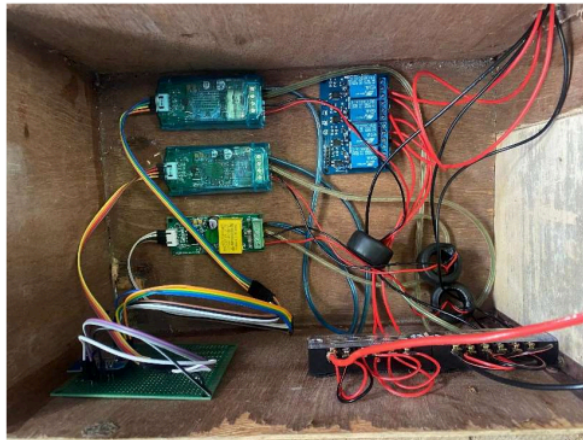
Gambar 11 Bagian Dalam Box Project
