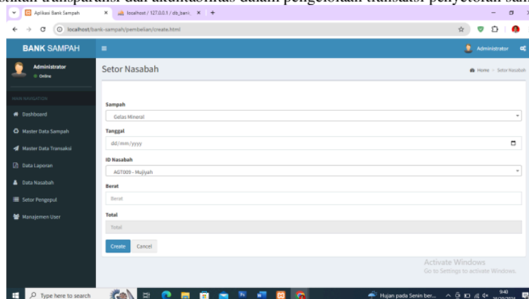
Gambar 5. Tambah Tabungan
