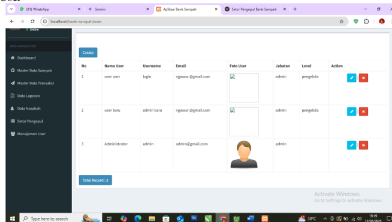
Gambar 7. Manajemen user
