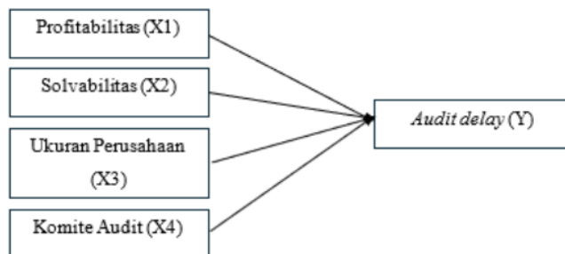
Gambar 2. Kerangka Konseptual
